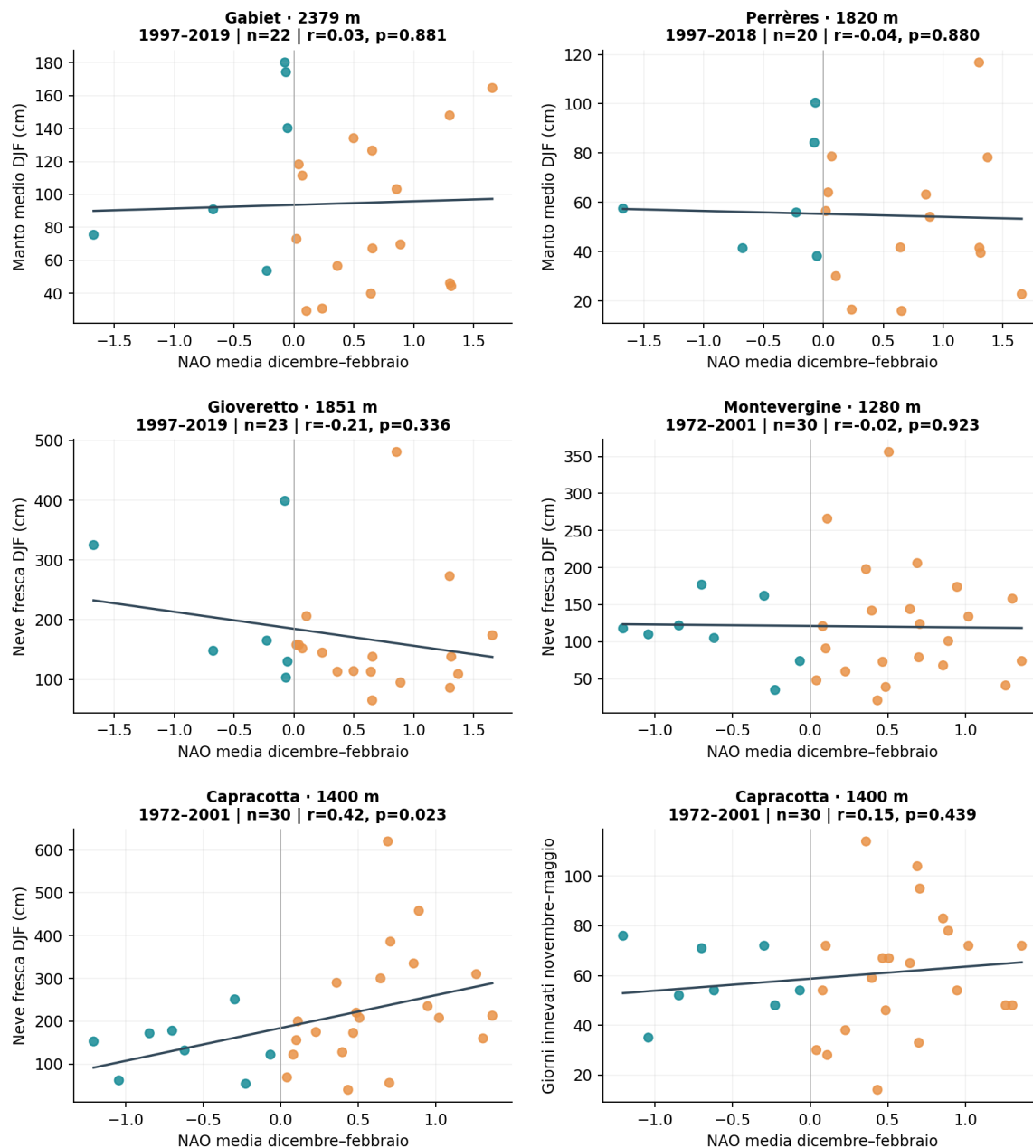
Figura 2. Ogni punto una stagione valida; azzurro = NAO, arancione = NAO+. Retta OLS descrittiva. Valori p nominali: tutti i test mostrati hanno q_{BH} > 0.05 . I primi tre pannelli riguardano il periodo recente parziale; gli ultimi tre il 1972-2001. Non un confronto su un trentennio comune recente. Fonti dati [1-3].
