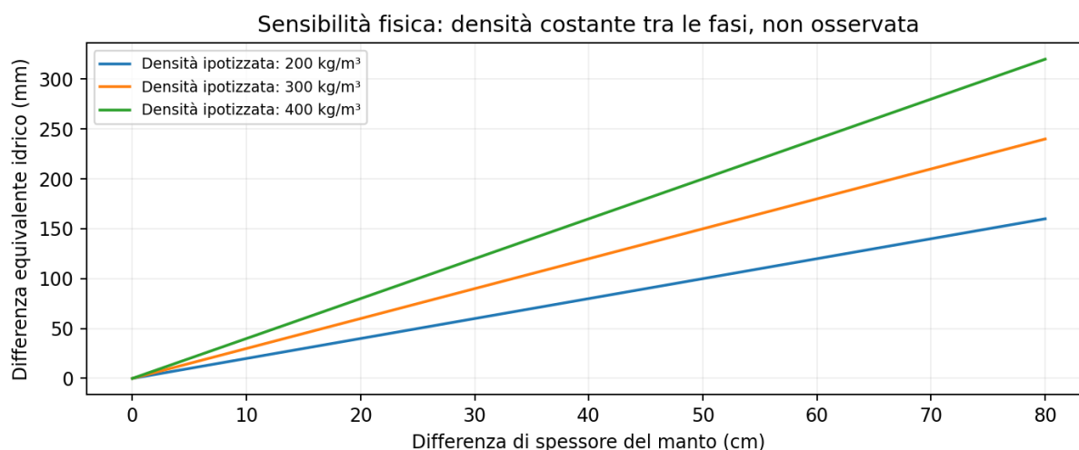
Figura 5. Scenari di densità scelti per illustrare la sensibilità. Per un confronto reale occorre calcolare separatamente HS e densità delle due fasi: SWE = (HS_{-} \cdot \text{densità}_{-} - HS_{+} \cdot \text{densità}_{+}) / 100 .
